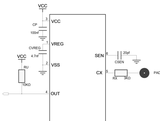
简化原理图
