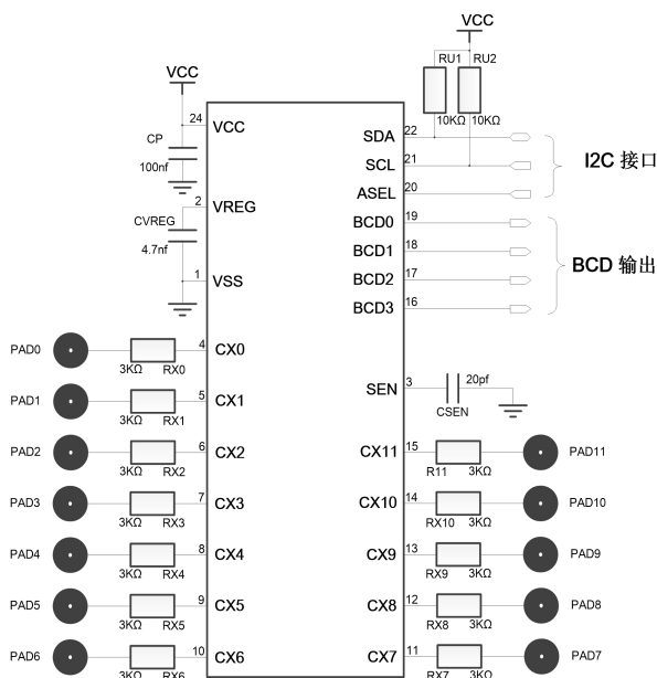
简化原理图
