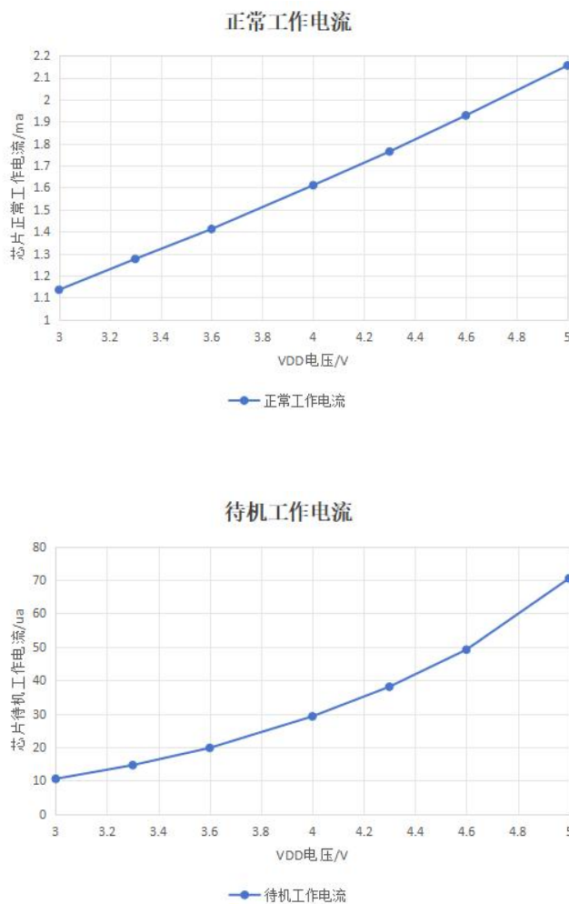
功耗情况（3~5V）
