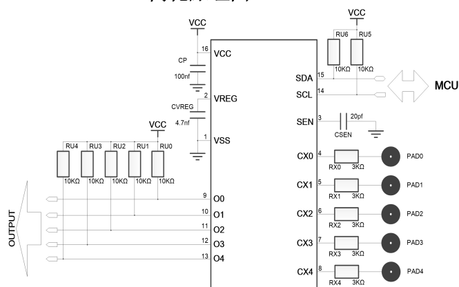
简化原理图
