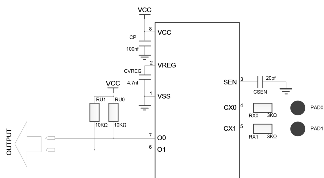
简化原理图
